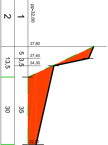
Przekrój 1+67.5
