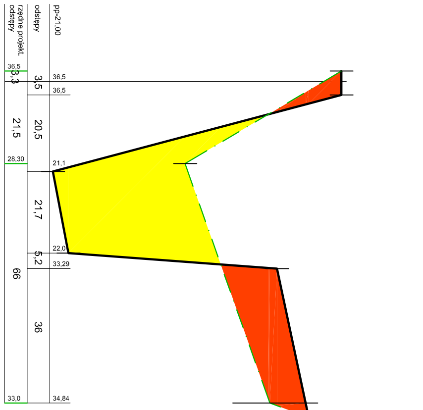
Przekrój 1+30.5
