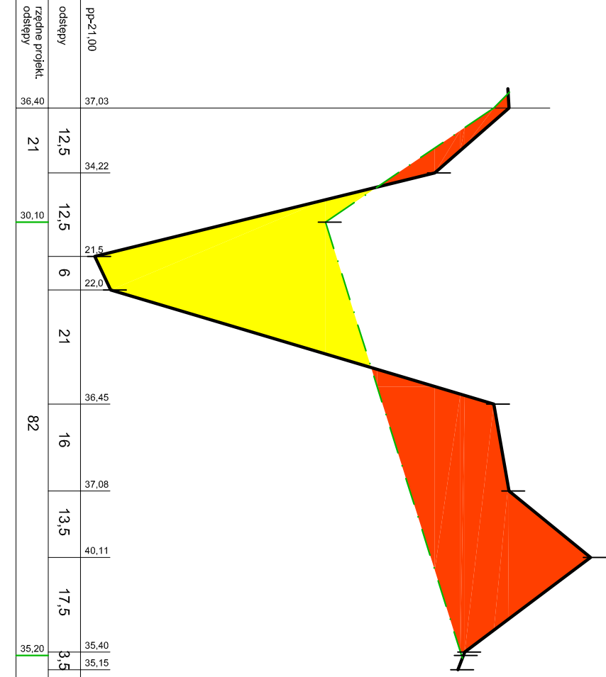
Przekrój 0+99.0
