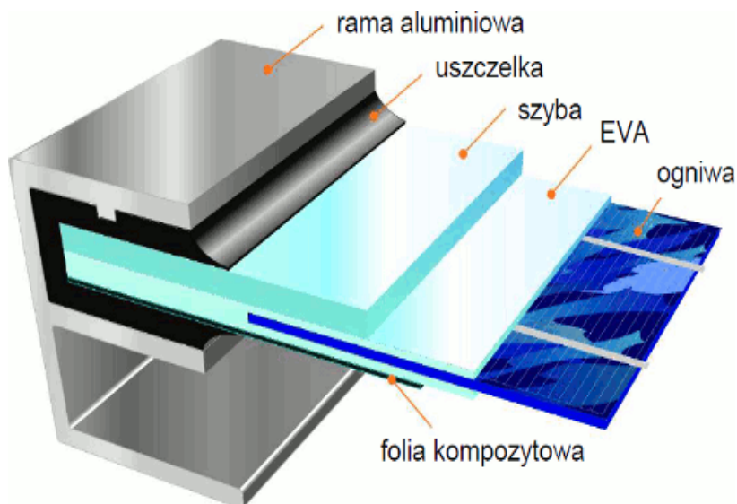
Rys nr 3. Budowa panelu fotowoltaicznego
