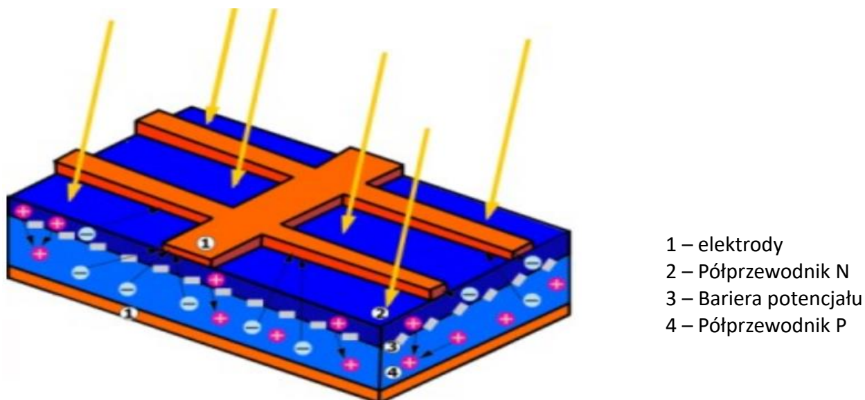
Rys nr 1. Budowa i sposób działania ogniwa fotoelektrycznego
